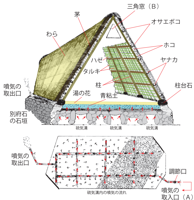
湯の花小屋のしくみモデル
