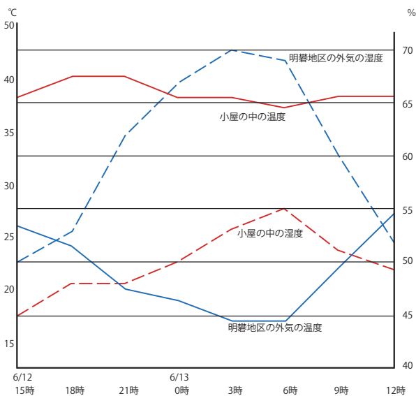
湯の花小屋の温度と湿度の変化
